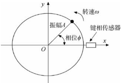
图 8 测试坐标定义示意图 Fig. 8 Measuring coordinate definition diagram
