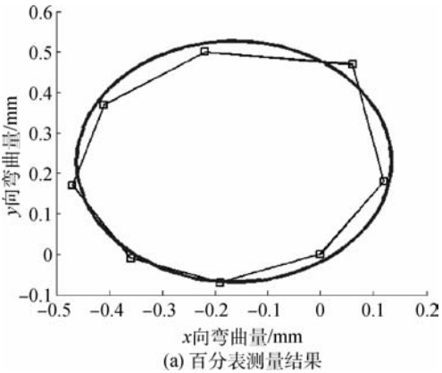
图 17 截面 1 结果 Fig. 17 Results of section 1
