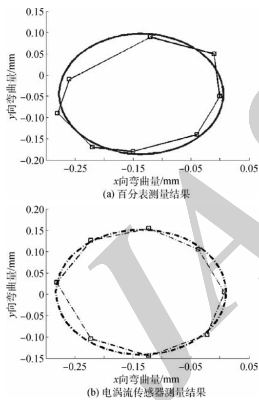
图 19 截面 3 结果 Fig. 19 Results of section 3
