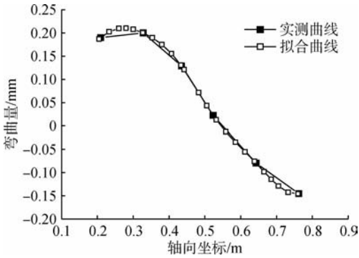
图 11 y 向转子弯曲曲线
