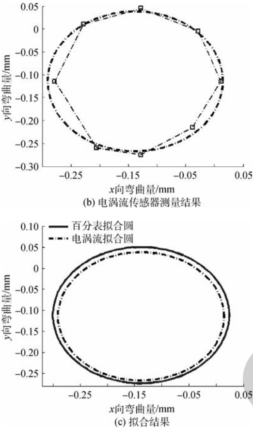
图 22 截面 6 结果 Fig. 22 Results of section 6
