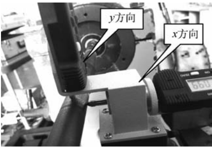
图 14 百分表测量转子弯曲局部放大图
