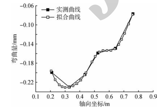
图 10 x 向转子弯曲曲线
