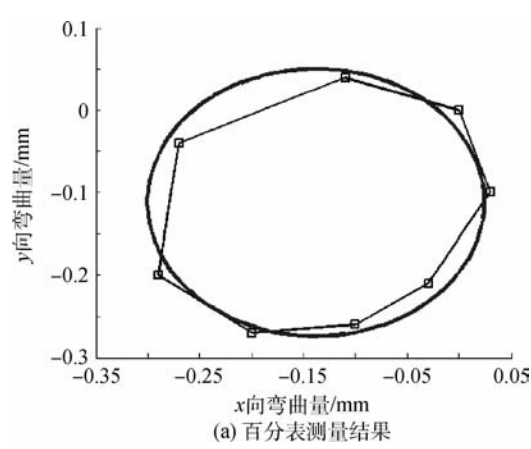
图 21 截面 5 结果 Fig. 21 Results of section 5
