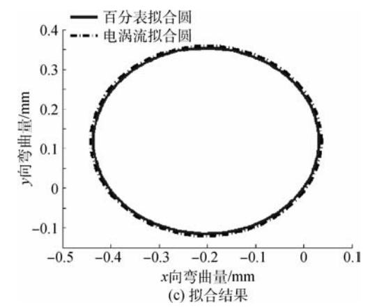
图 19 截面 3 结果 Fig. 19 Results of section 3
