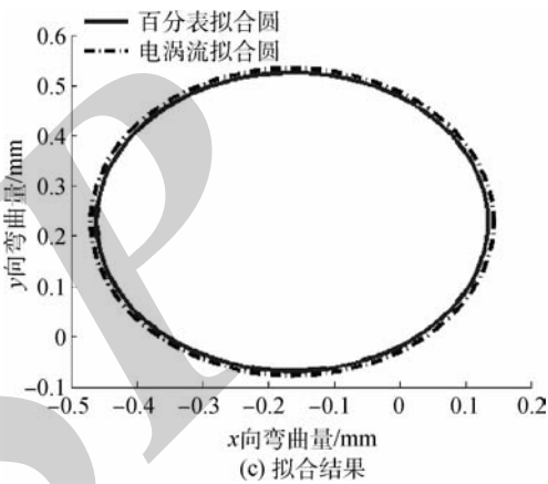
图 18 截面 2 结果 Fig. 18 Results of section 2
