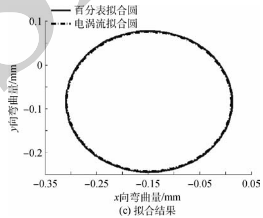
图 21 截面 5 结果 Fig. 21 Results of section 5
