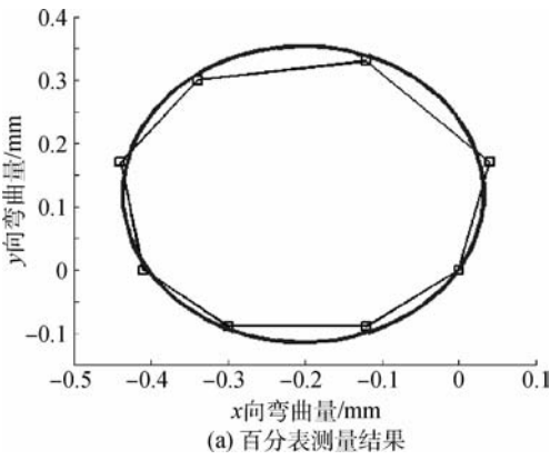
图 18 截面 2 结果 Fig. 18 Results of section 2
