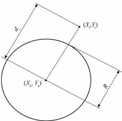
图 16 最小二乘法拟合圆心
